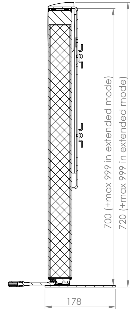
SECTION B-B SCALE 1 : 5
