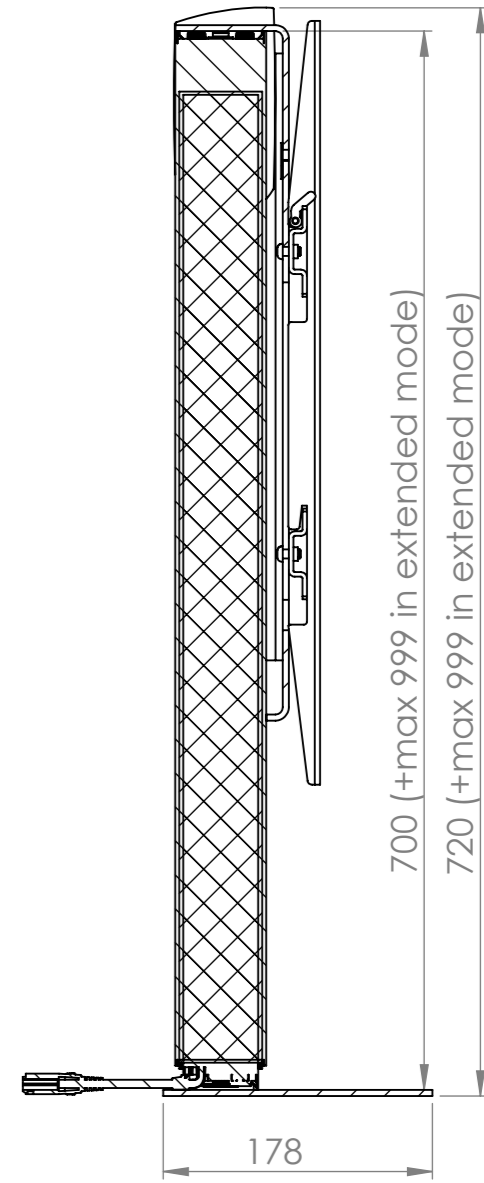
SECTION B-B SCALE 1 : 5
