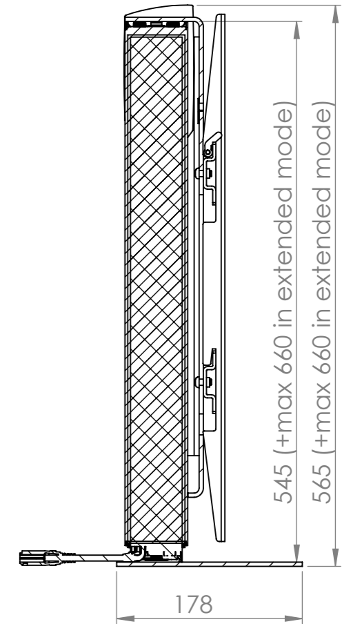
SECTION B-B SCALE 1 : 5
